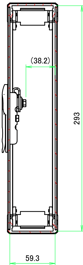
B-B ( 1 : 3 )
