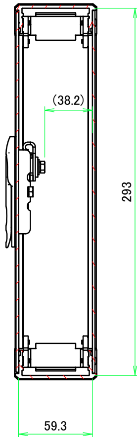
B-B ( 1 : 3 )
