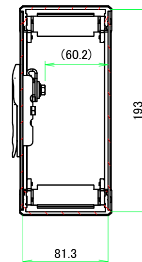
B-B ( 1 : 3.5 )
