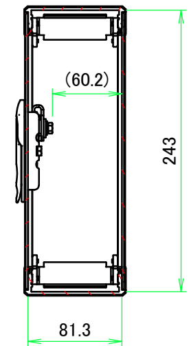
B-B ( 1 : 4.5 )
