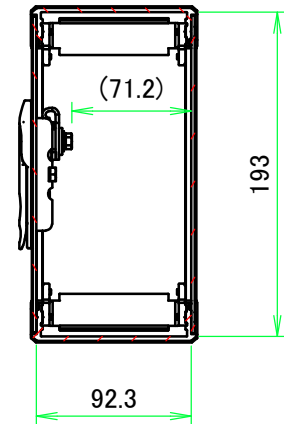
B-B ( 1 : 4.5 )
