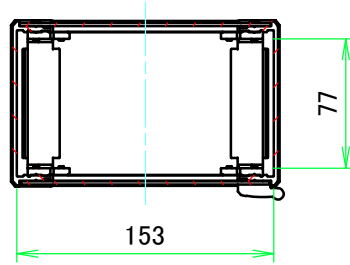
A-A ( 1 : 4.5 )
