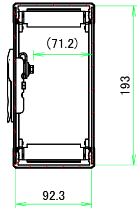
B-B ( 1 : 4.5 )
