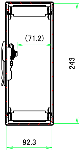
B-B ( 1 : 4.5 )
