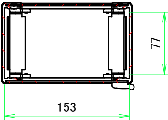
A-A ( 1 : 4.5 )
