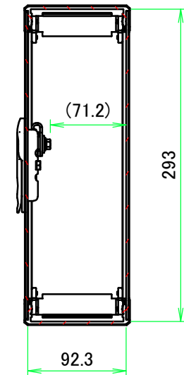
B-B ( 1 : 5 )
