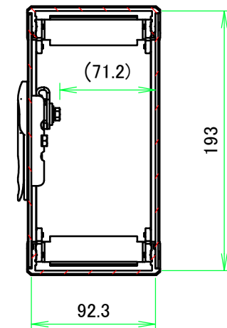
B-B ( 1 : 4 )
