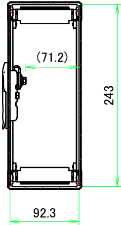
B-B ( 1 : 5 )
