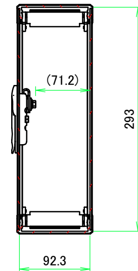
B-B ( 1 : 5 )
