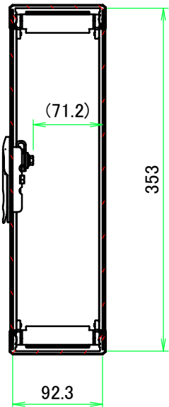
B-B ( 1 : 5.5 )
