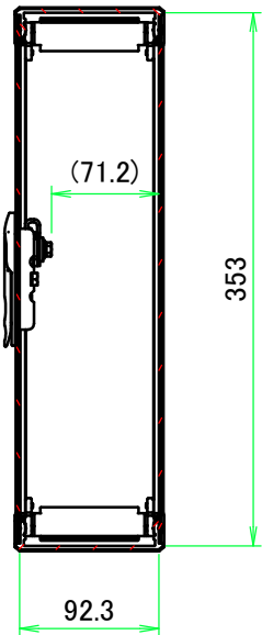
B-B ( 1 : 5.5 )
