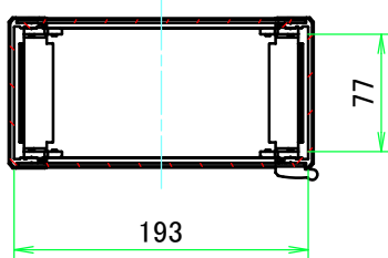
A-A ( 1 : 5.5 )
