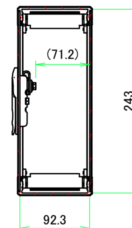
B-B ( 1 : 5 )
