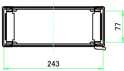
A-A ( 1 : 5.5 )
