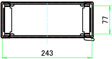
A-A ( 1 : 6 )
