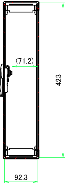
B-B ( 1 : 6 )
