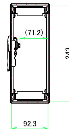
B-B ( 1 : 5.5 )
