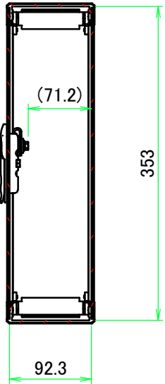
B-B ( 1 : 6 )
