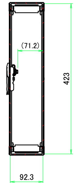
B-B ( 1 : 6.5 )
