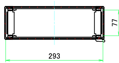
A-A ( 1 : 6.5 )
