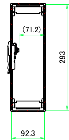
B-B ( 1 : 6.5 )
