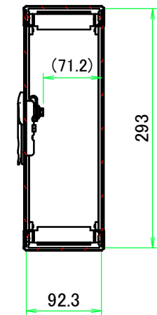
B-B ( 1 : 6.5 )
