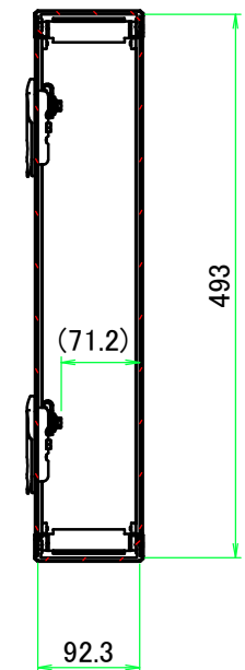
B-B ( 1 : 7.5 )
