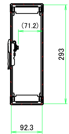
B-B ( 1 : 6.5 )
