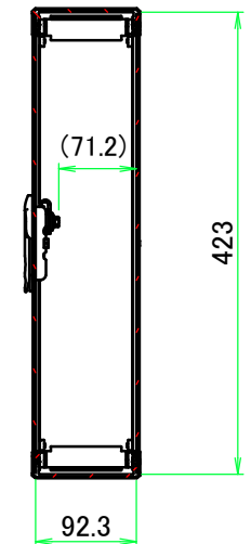
B-B ( 1 : 7.5 )
