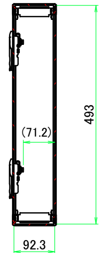
B-B ( 1 : 8.5 )
