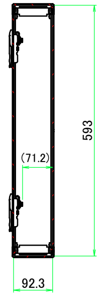
B-B ( 1 : 9 )
