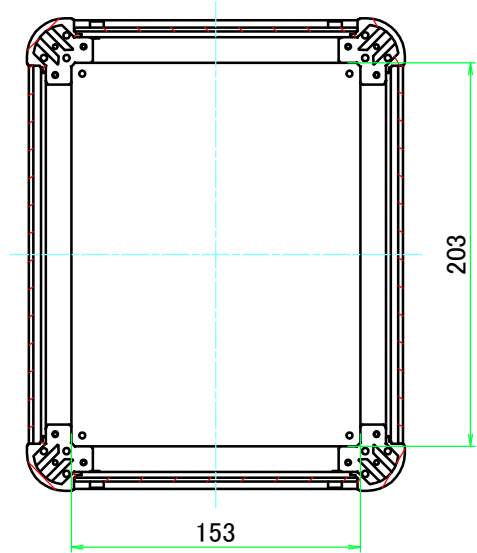
B-B ( 1 : 4 )
