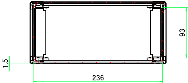
A-A ( 1 : 4 )
