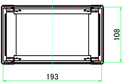
C-C ( 1 : 4.5 )
