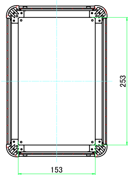
B-B ( 1 : 4.5 )
