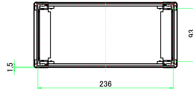
A-A (1:4)
