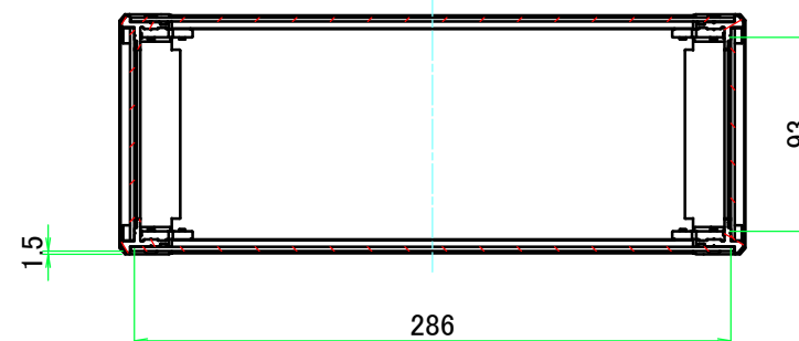
A-A (1:4)
