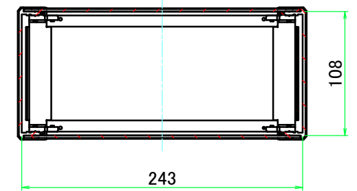
C-C ( 1 : 4.5 )
