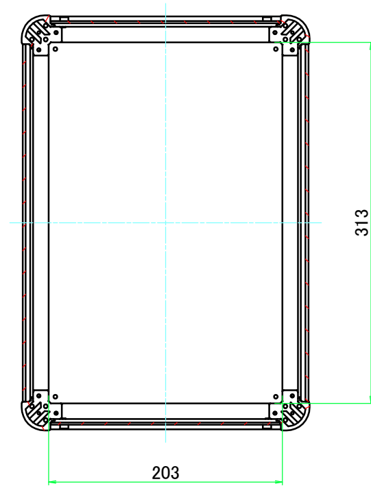
B-B ( 1 : 4.5 )
