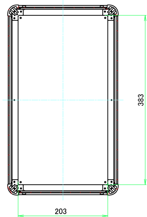
B-B ( 1 : 5 )
