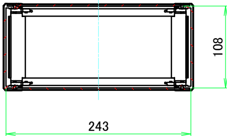
C-C ( 1 : 5 )
