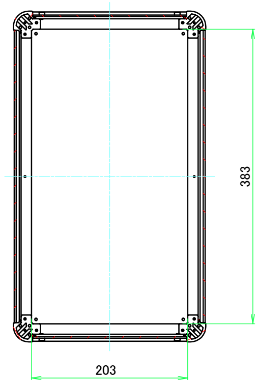
B-B ( 1 : 5 )
