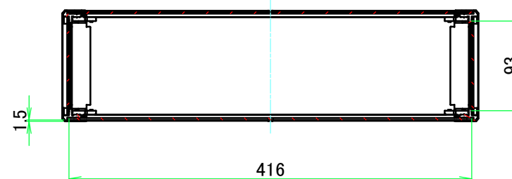
A-A ( 1 : 5.5 )
