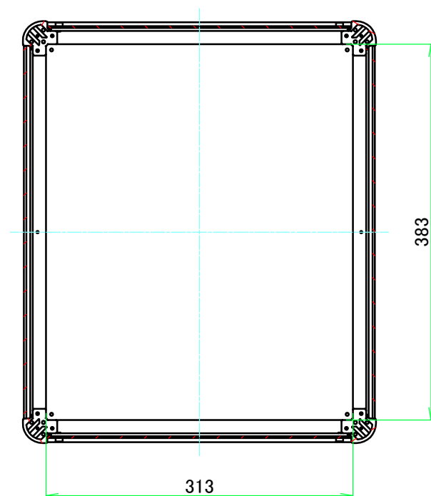
B-B ( 1 : 5.5 )
