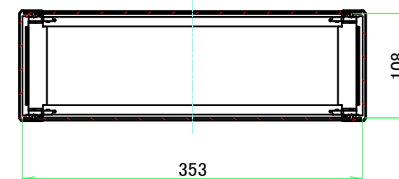
C-C ( 1 : 5.5 )
