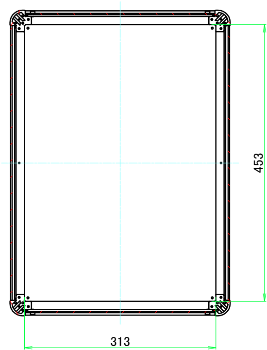
B-B ( 1 : 6 )
