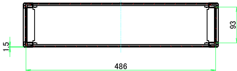
A-A ( 1 : 6 )
