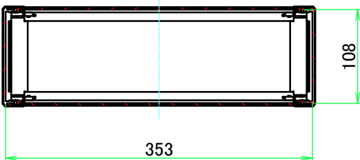
C-C ( 1 : 6 )
