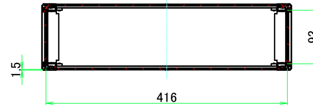
A-A ( 1 :6.5 )
