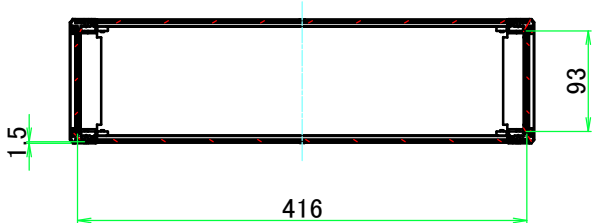
A-A ( 1 : 7 )
