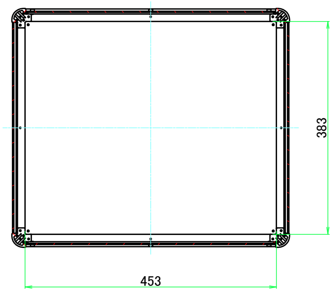
B-B ( 1 : 7 )
