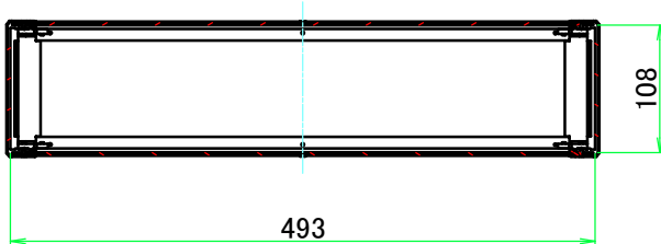
C-C ( 1 : 7 )
