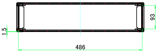
A-A ( 1 : 7 )
