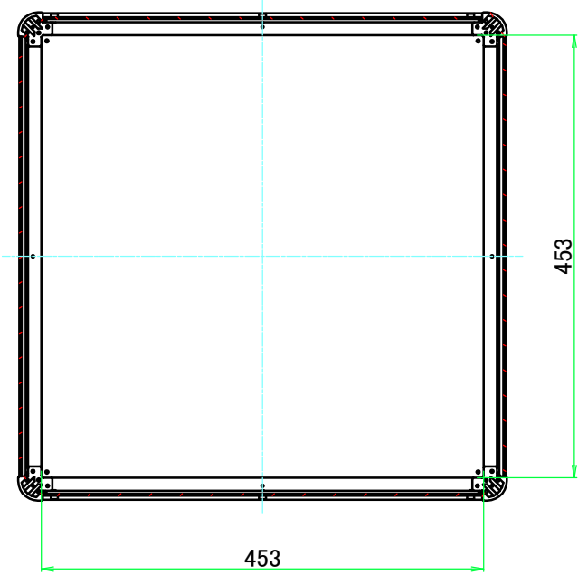
B-B ( 1 : 7 )
