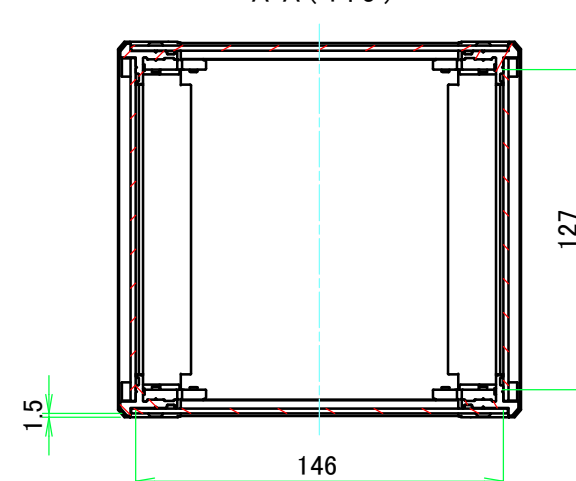
A-A (1:3)
