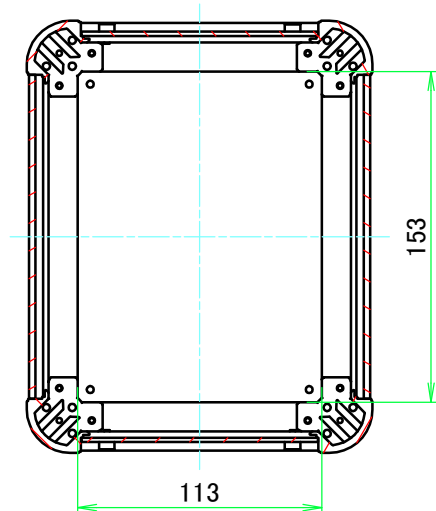
B-B ( 1 : 3.5 )
