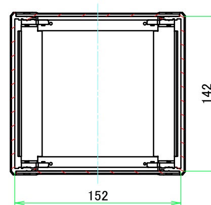
C-C ( 1 : 3.5 )
