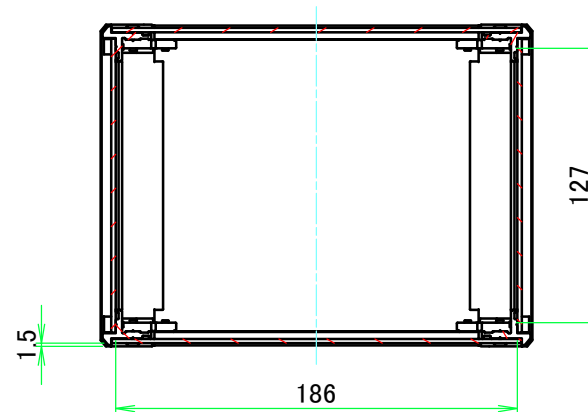
A-A ( 1 : 3.5 )
