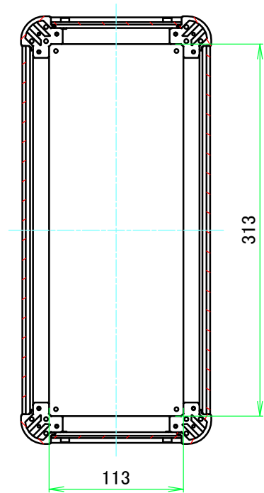
B-B ( 1 : 4.5 )
