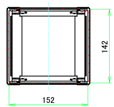
C-C ( 1 : 4.5 )
