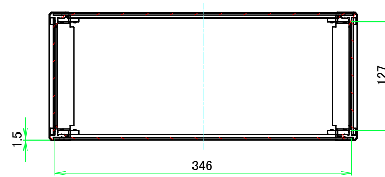
A-A ( 1 : 4.5 )
