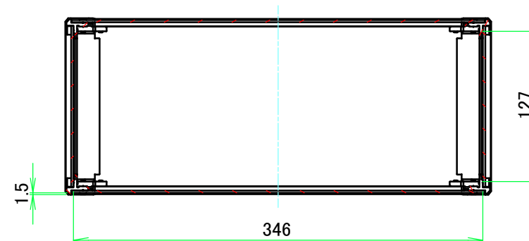
A-A ( 1 : 4.5 )
