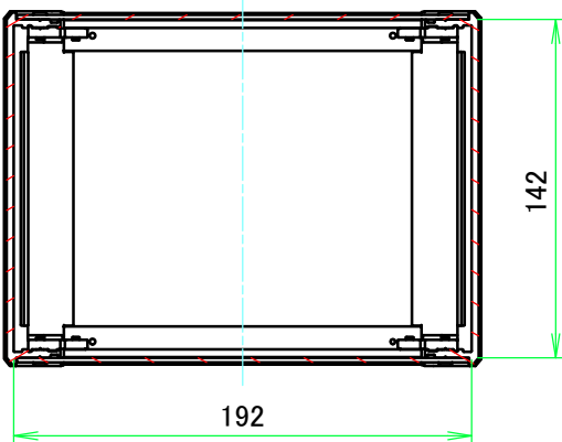
C-C ( 1 : 3.5 )
