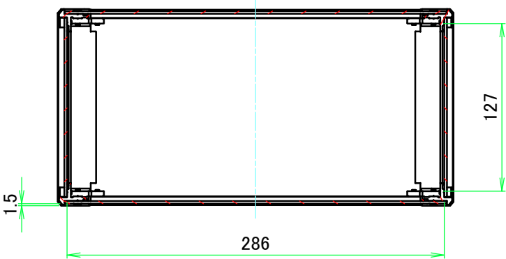
A-A ( 1 : 4 )
