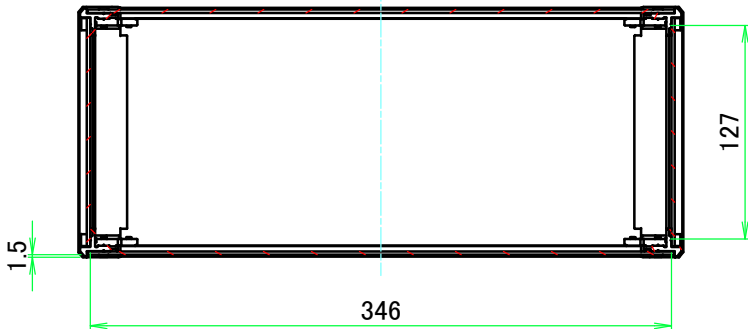
A-A ( 1 : 4.5 )
