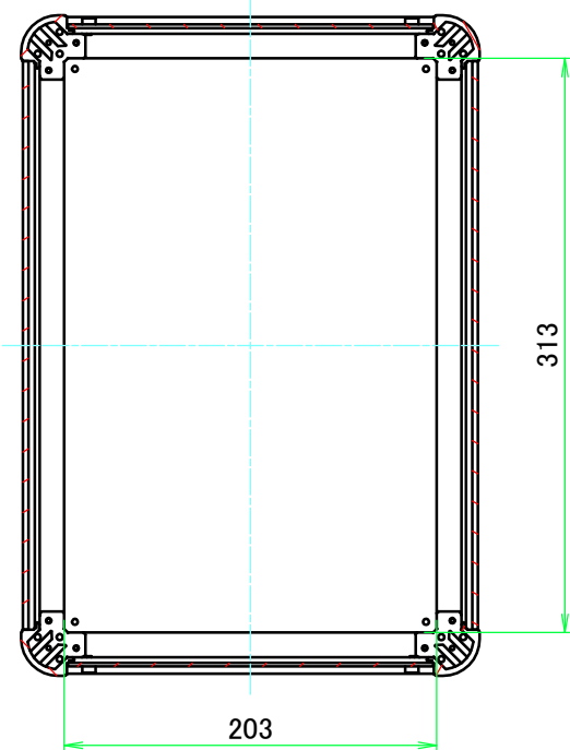
B-B ( 1 : 4.5 )
