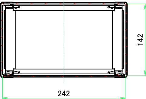
C-C ( 1 : 4.5 )
