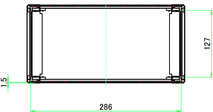
A-A ( 1 : 4.5 )
