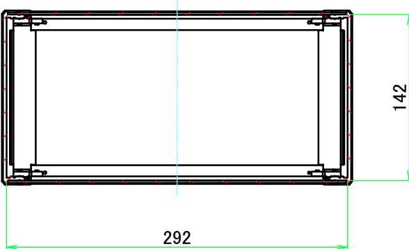
C-C ( 1 : 4.5 )
