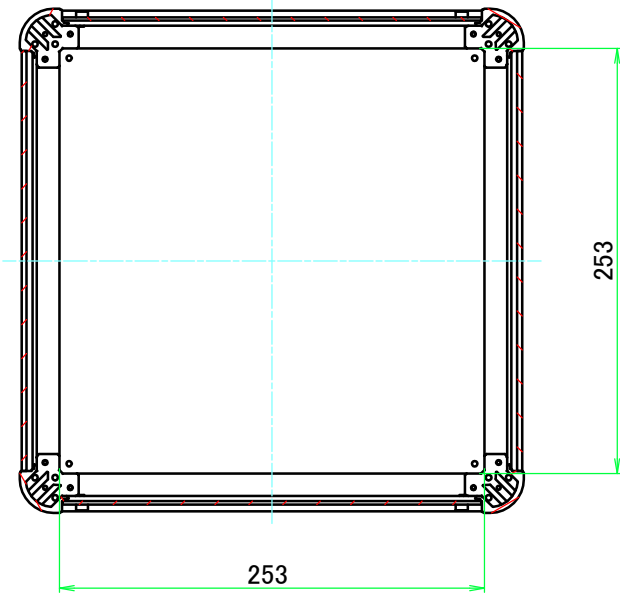
B-B ( 1 : 4.5 )
