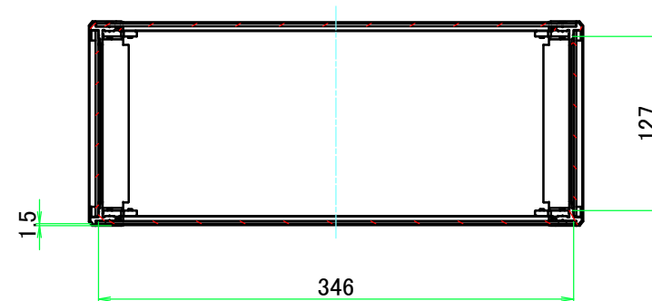
A-A (1:5)
