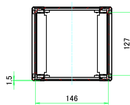
A-A ( 1 : 4.5 )
