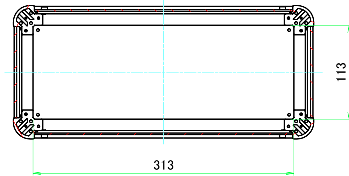
B-B ( 1 : 4.5 )
