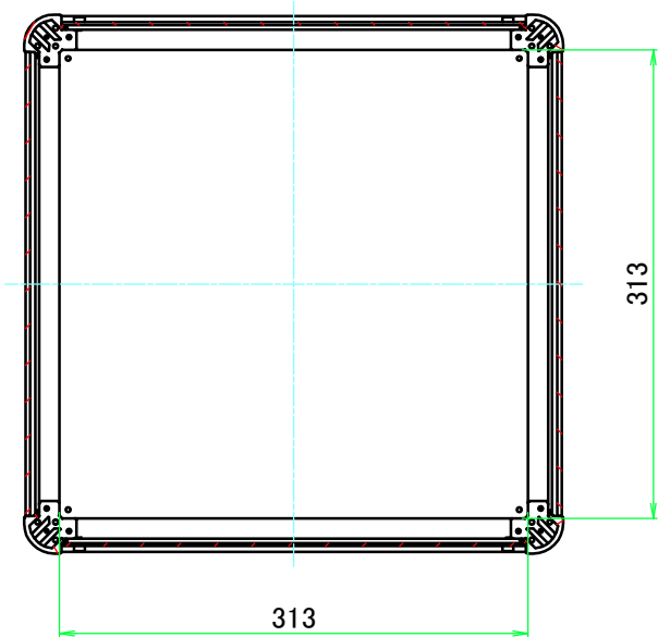
B-B ( 1 : 5.5 )
