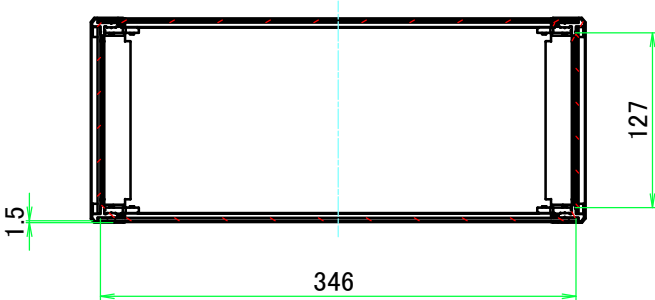
A-A ( 1 : 5.5 )
