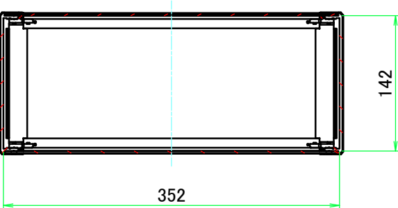
C-C ( 1 : 5.5 )
