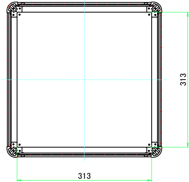
B-B ( 1 : 5.5 )
