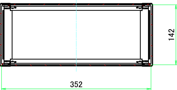
C-C ( 1 : 5.5 )
