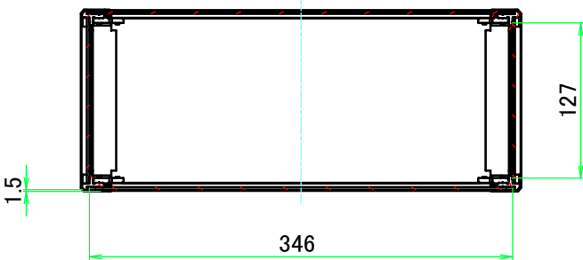
A-A ( 1 : 5.5 )
